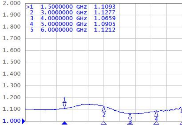
图1.合路端驻波比
